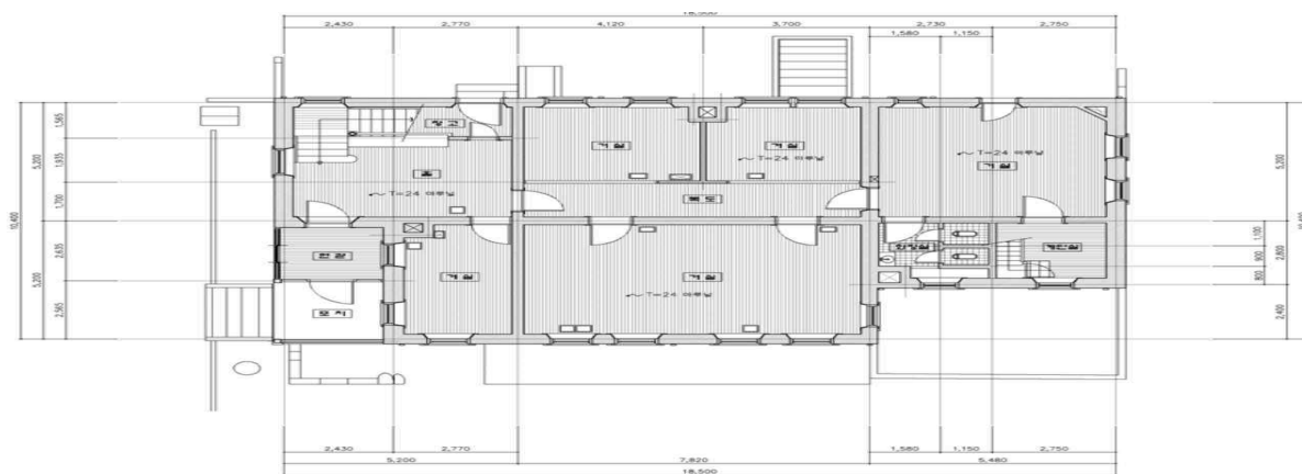
1층 평면도
